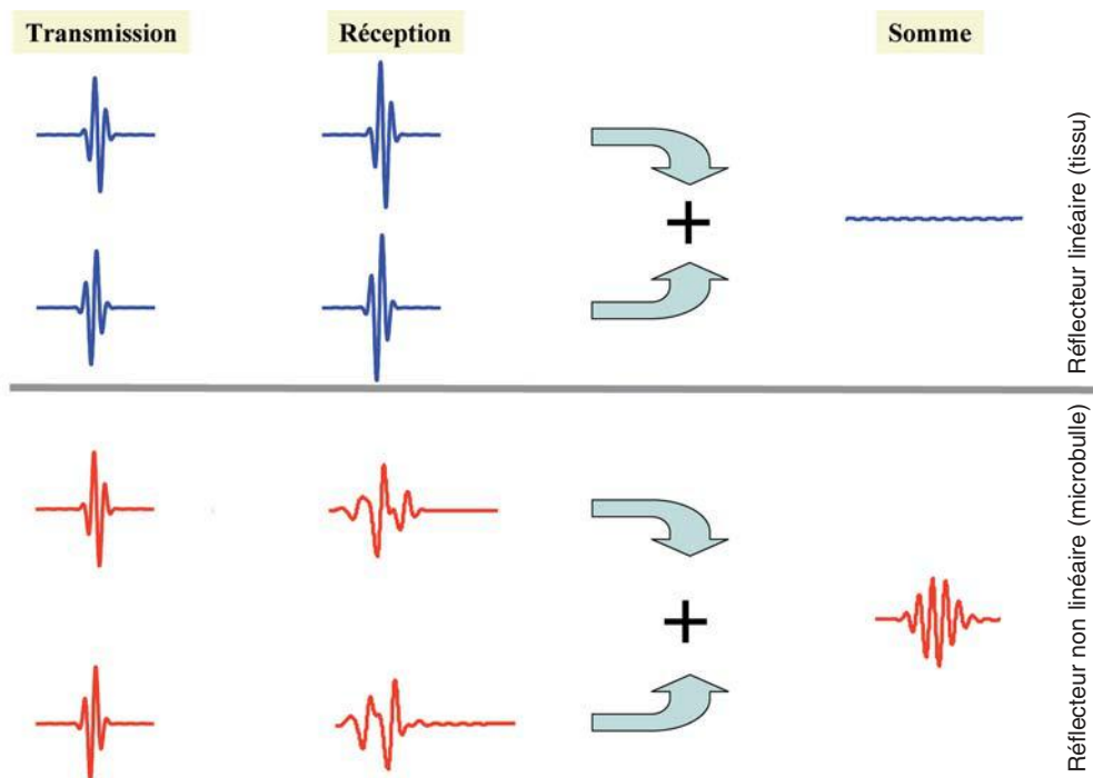
Fig. 7 - Principe de l'imagerie par inversion de phases.
