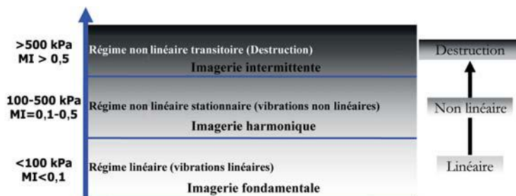
Fig. 2 - Régimes acoustiques de la microbulle en fonction de l'index mécanique.
