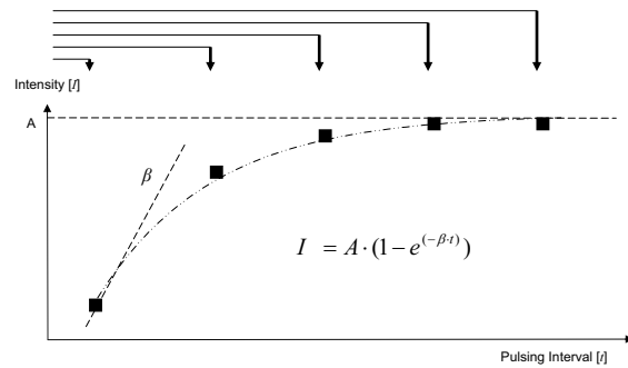
Fig. 4 - Cinétiques de remplissage. Diagramme schématisant les cinétiques de remplissage à IM élevé avec des intervalles de temps croissants. Après la destruction des bulles par une impulsion ultrasonore destructrice, un intervalle croissant entre deux impulsions ultrasonores conduit à une augmentation du degré de remplissage de la région par les bulles entre deux impulsions qui peut être détecté en tant qu'augmentation du signal. L'interval de pulsation résultant peut être évalué par un modèle exponentiel. I = \text{intensité} , A = \text{plateau de l'intensité l'écho} , \beta = \text{taux constant déterminant le taux d'augmentation de l'intensité de l'écho} , t = \text{interval de pulsation} .
