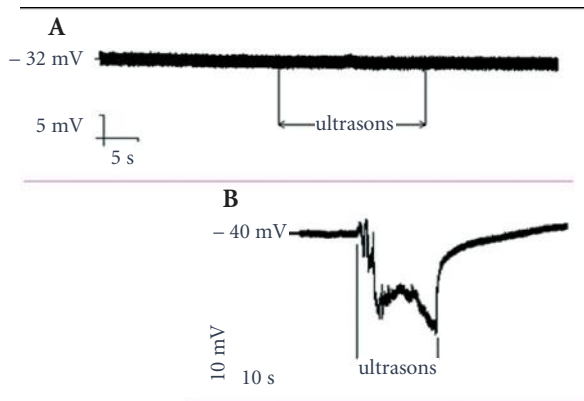
Fig. 5 - Potentiel membranaire d'une cellule MDA-Mb231 sous l'effet des ultrasons (200 kPa, 1 MHz) seul (A) et en présence d'ultrasons (200 kPa, 1 MHz) et microbulles de SonoVue® (B).
